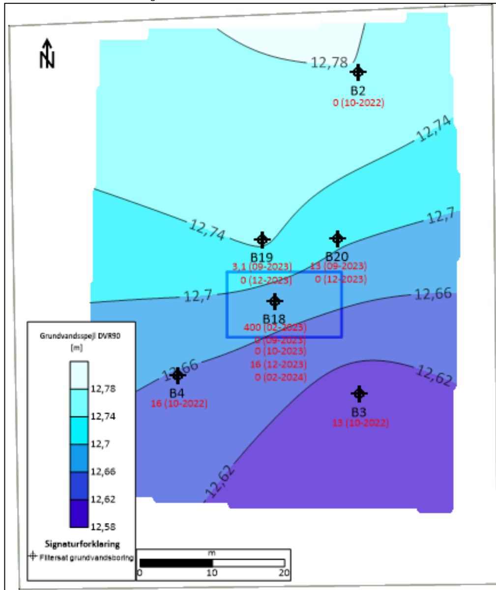
Figur 1 Potentialekort september 2023. Med rødt anvist totalkulbrinter, urensset \mu\text{g/l} efterfulgt af prøvetagningsmåned. Blå firkant indikerer V1-kortlagte areal. Surfer fra Golden Software
